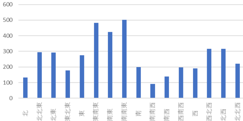
方角別風向
