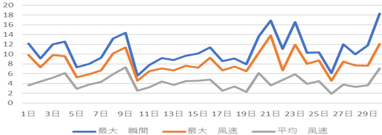
最大風速・最大瞬間風速・平均風速
