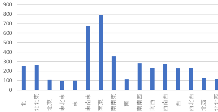
風向頻度
