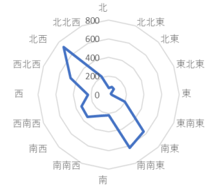
風向頻度レーダーチャート
